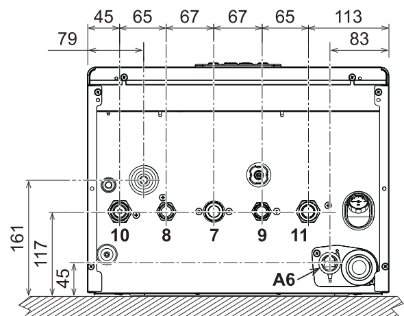
Vista inferior
