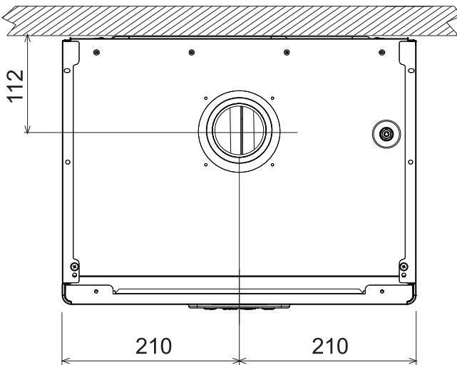
Vista superior
